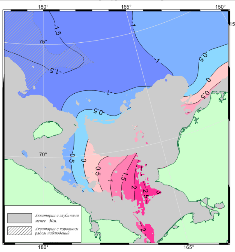
Распределение Температуры (°C) на горизонте 50м, лето
